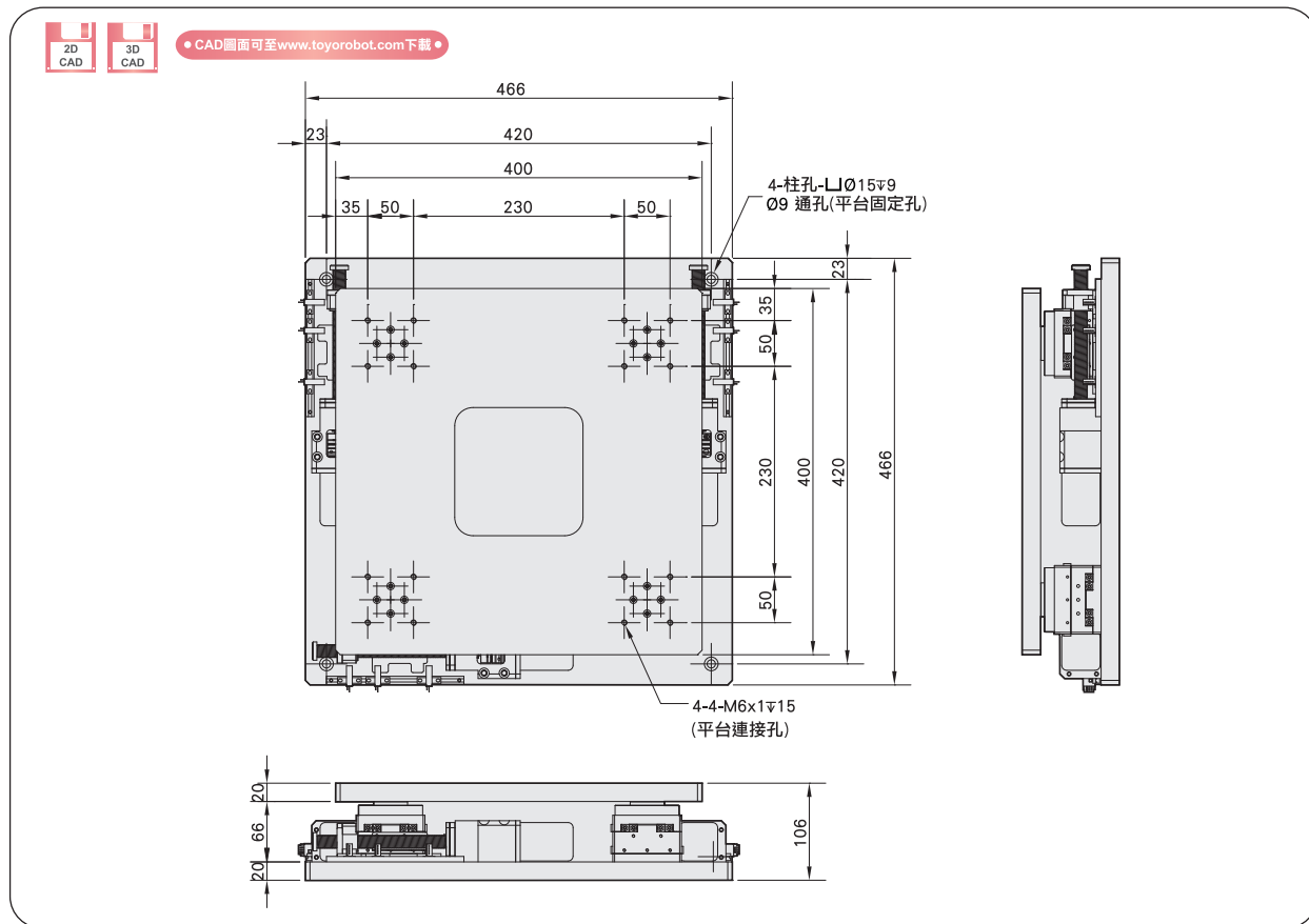
EXYY-040-040-42M 尺寸圖 Size
