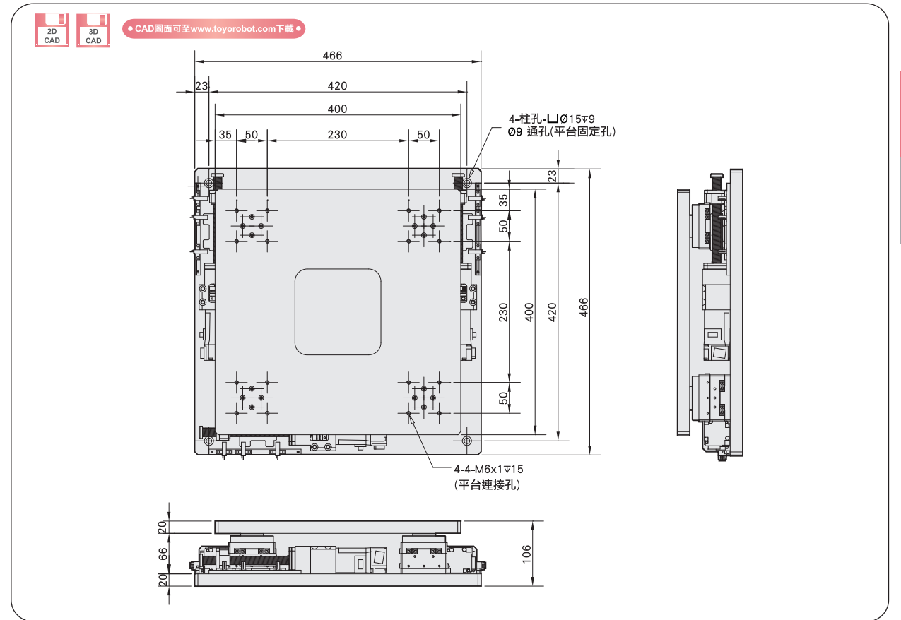
EXYY-040-040-M10 尺寸圖 Size
